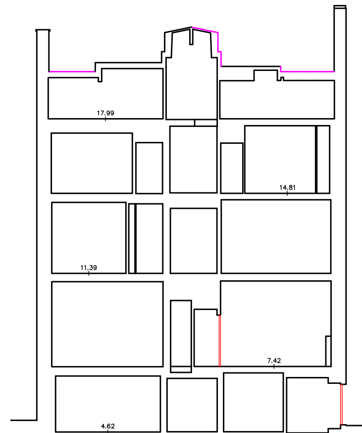
Section D-D
